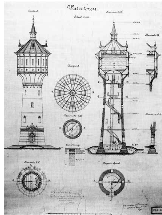
Revisieschets van de Watertoren aan de Wierdensestraat eind 1800
